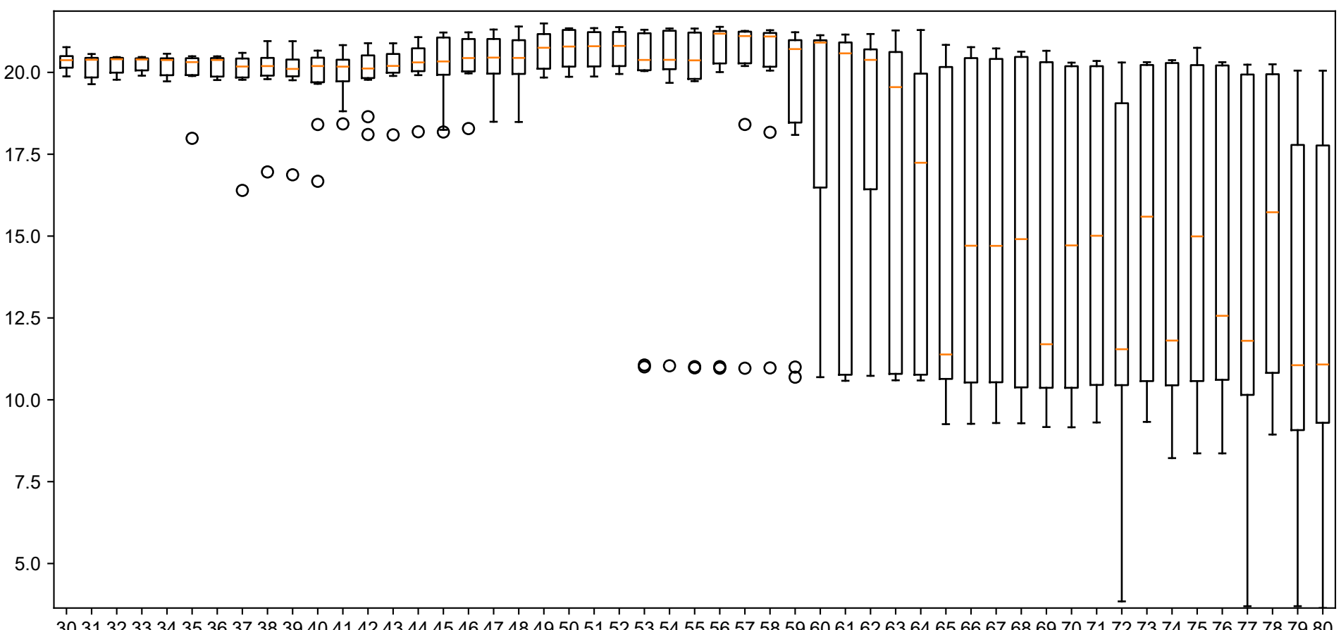
nn
