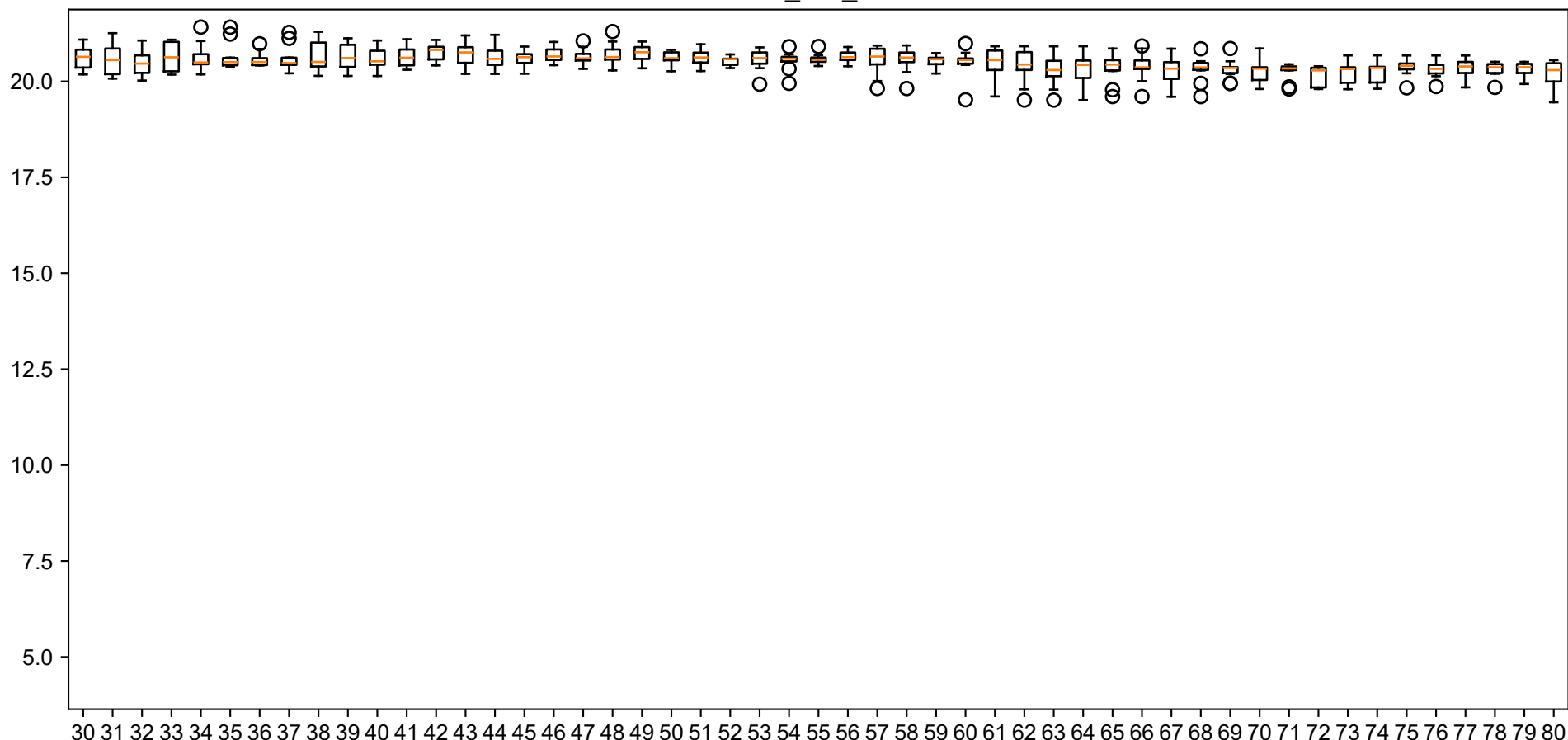
elastic_net
