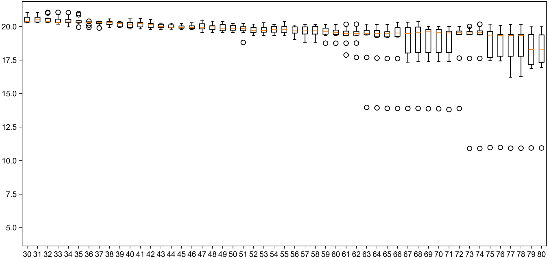
lasso
